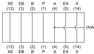
PORT 4
